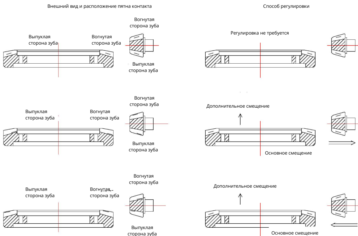
Рис. 4-23. Пятно контакта
