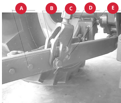
Рис. 2-71. Нижняя тяга
