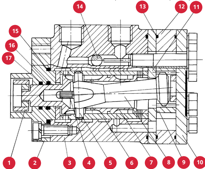
Рис. 4-28. Рулевой механизм
