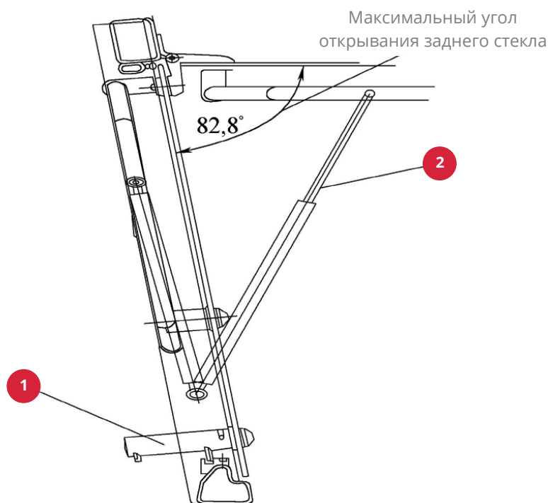
Рис. 2-49. Заднее стекло
