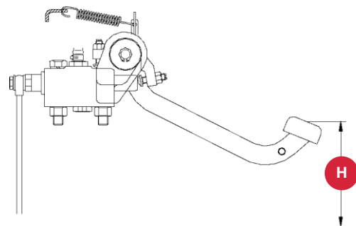
Рис. 4-34-3. Педаль тормоза
