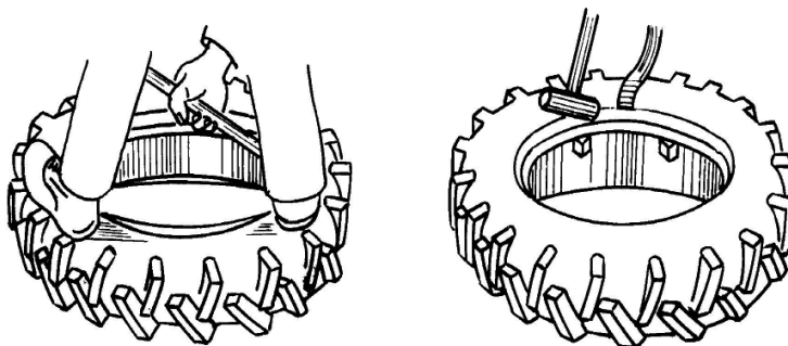
Рис. 2-36. Монтаж шины
