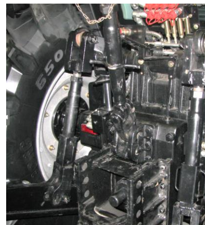
Рис. 2-52. Система подъема рабочего оборудования
