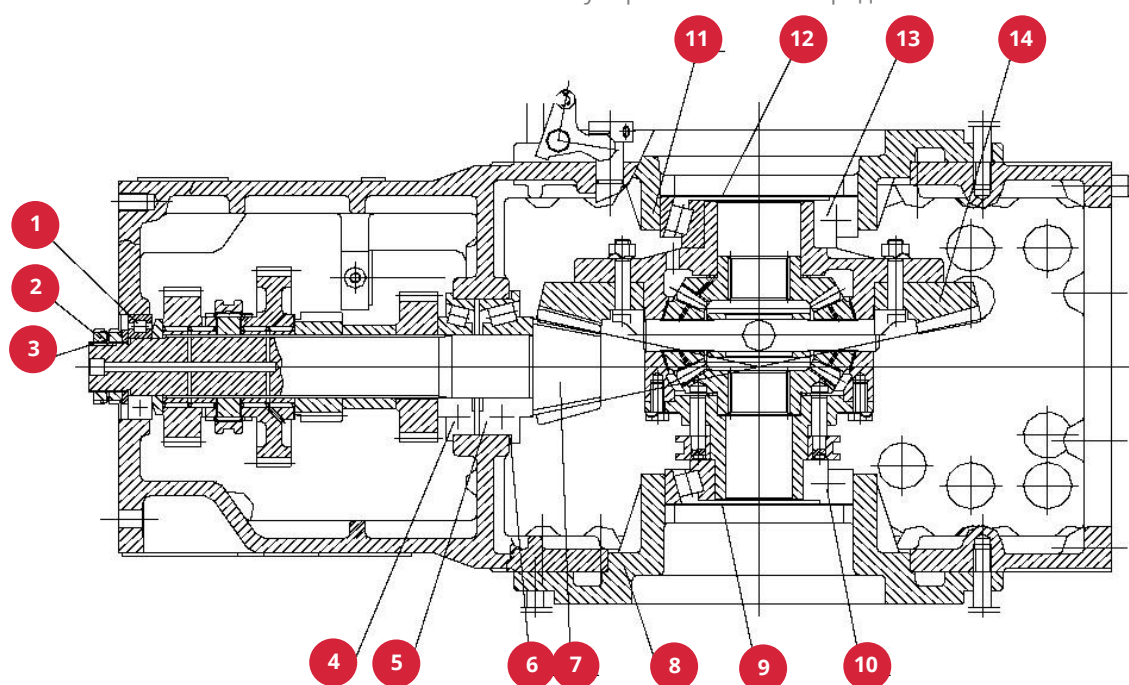
Рис. 4-22. Регулировка главной передачи
